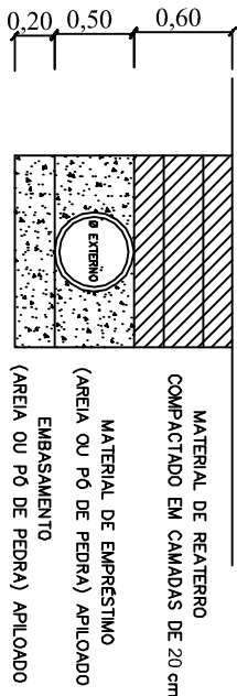
DETALHE DO ASSENTAMENTO DO TUBO 0,40M SEM ESCALA
