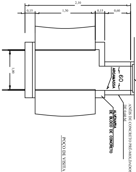
CORTE A-A SEM ESCALA
